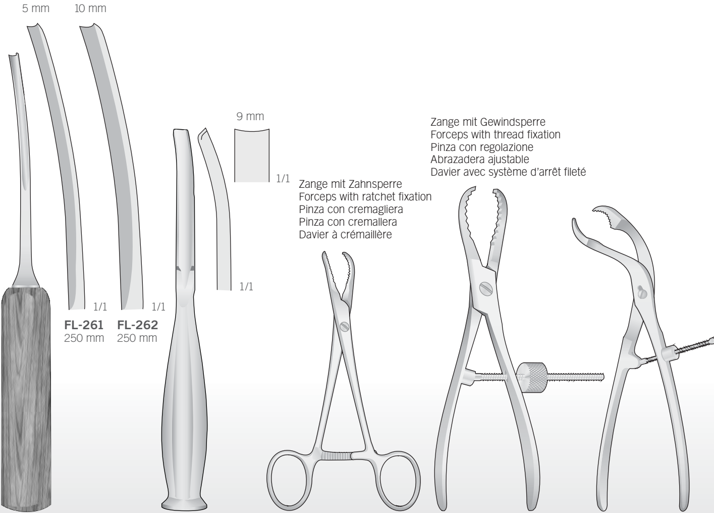
LEXER FL-261 250 mm
